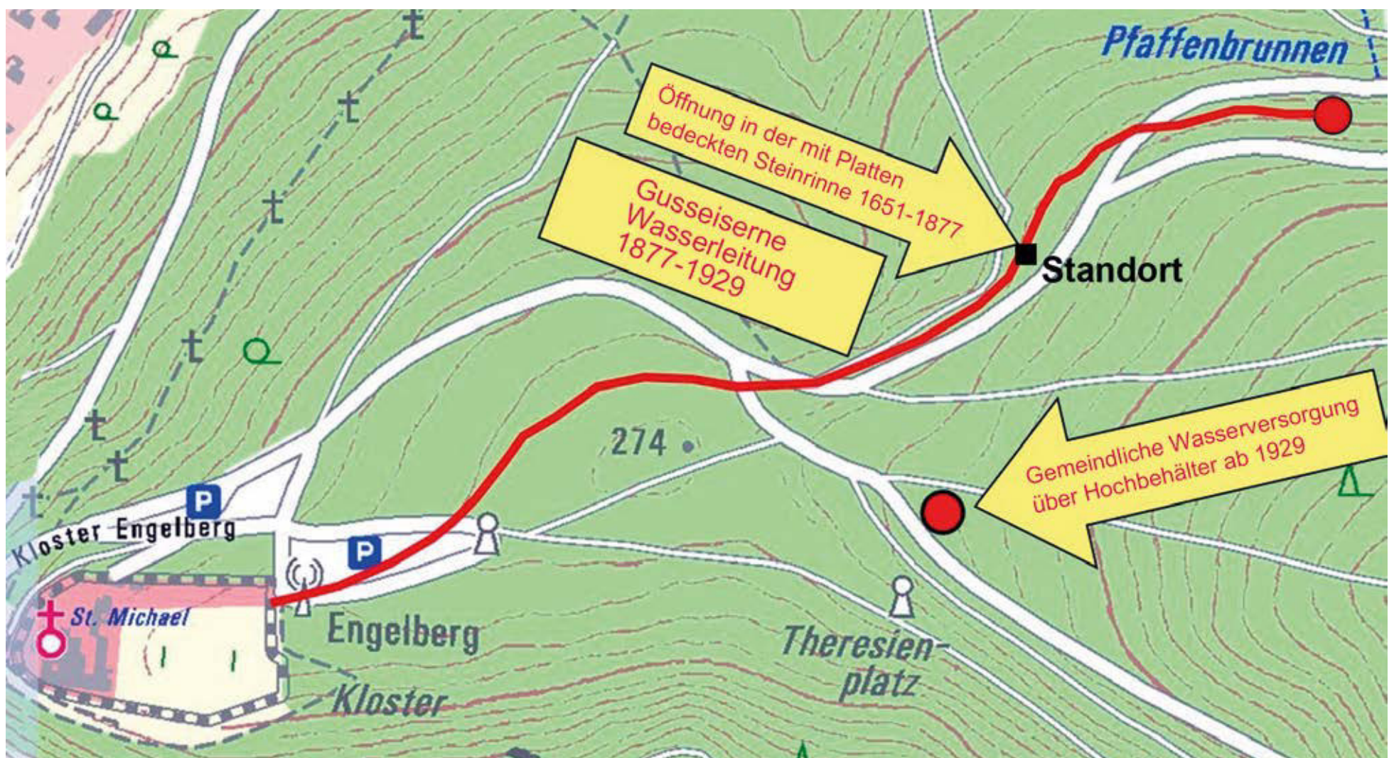
Plan der historischen Wasserversorgung des Klosters Engelberg durch den Pfaffenbrunnen bis 1929
